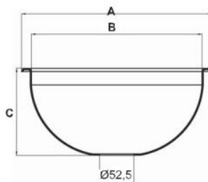
Cubas semiesféricas para encastrar en acero inoxidable.
