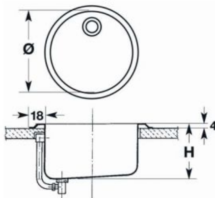
Cuba redonda para encastrar.
